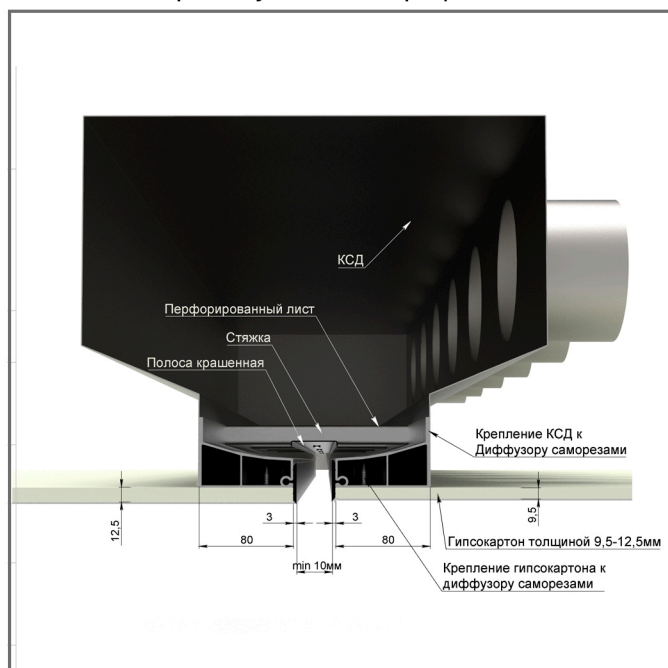
Вариант установки профиля
