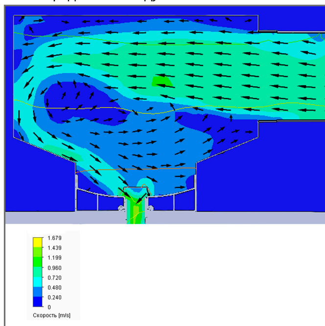
Распределение воздушного потока в сечении
